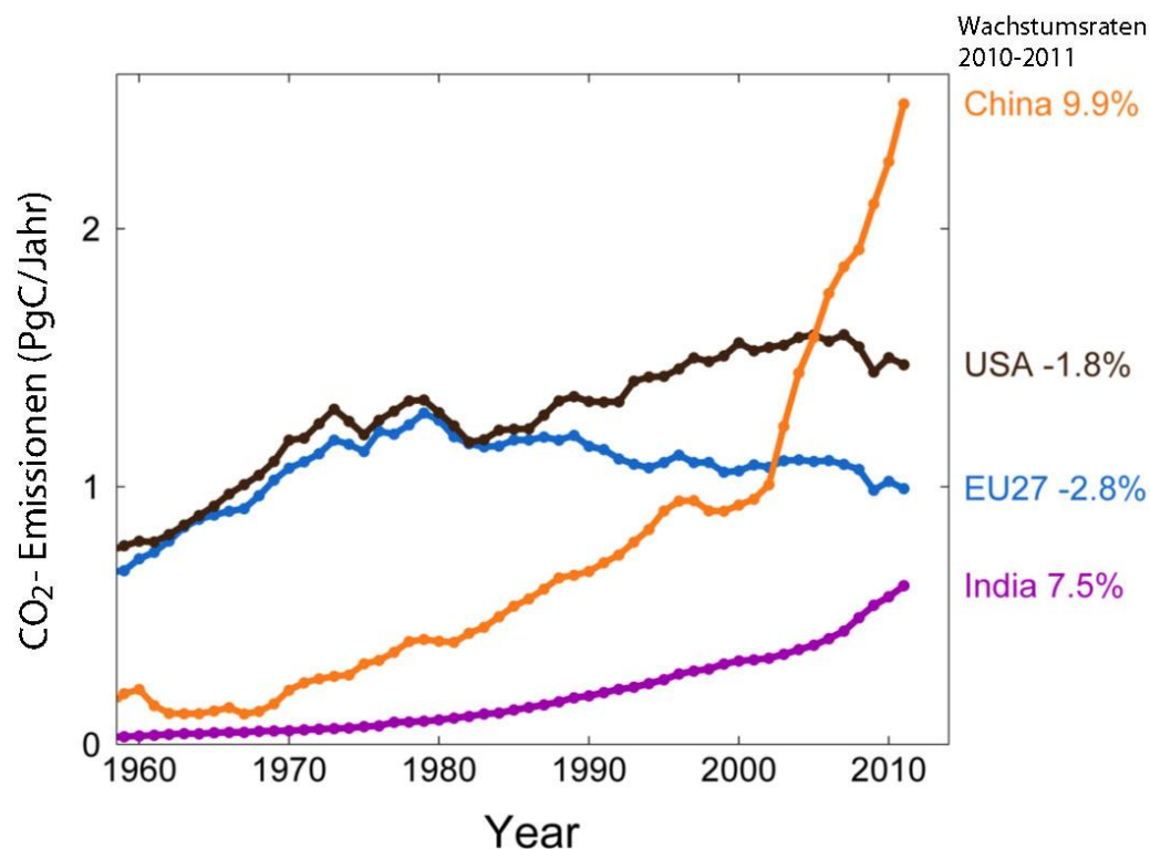
Bild: Jährliche Entwicklung der CO 2 -Emissionen in verschiedenen Ländern (Autor: C. LeQuéré)
